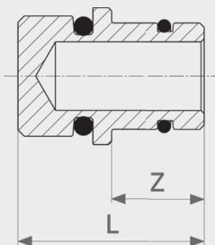
Соединительный элемент переходной - ! Модель 2233.6
