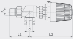
Угловой радиаторный вентиль - латунь никелированная Модель 1075.96
