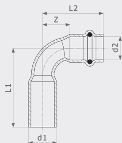
Отвод редуционный 90° Profipress - медь Модель 2416.2
