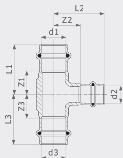
Тройник Sanpress - ! Модель 2218
