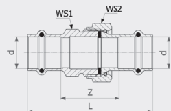
Соединительный элемент резьбовой Sanpress - ! Модель 2260
