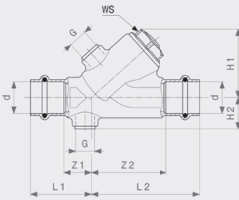
Обратный клапан Easytop Модель 2239
