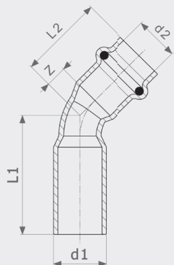
Отвод редуционный 45° Profipress - медь Модель 2426.2
