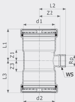
Тройник Profipress XL - медь Модель 2417.2XL
