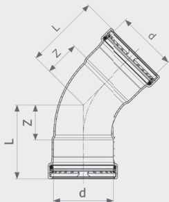
Отвод 45° Profipress XL - медь Модель 2426XL
