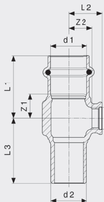
Тройник Sanpress, G \frac{1}{4} , с вставной муфтой - ! Модель 2217.4
