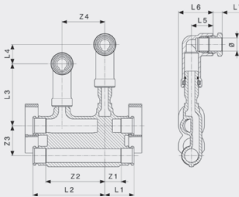
Подключение радиаторов при плинтусной разводке - бронза Модель 2277.2
